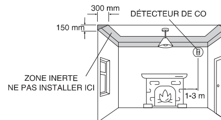
Figure 1: Installation dans une pièce avec chauffage brûlant du combustible
