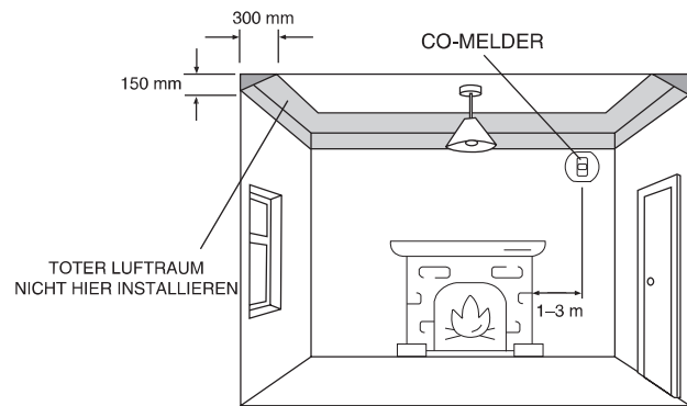
Abbildung 1: Installation in einem Raum mit einem Brennstoffverbrennungsgerät
